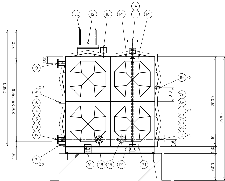
本体立面図
