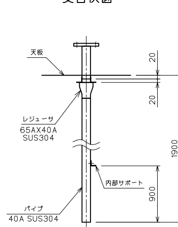
受台伏図
