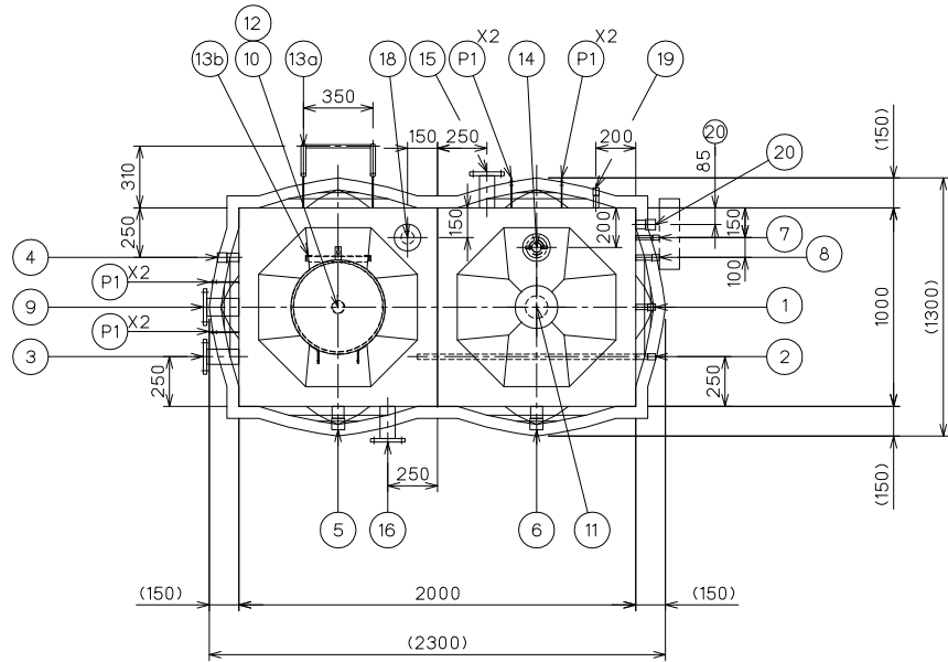
本体平面図
