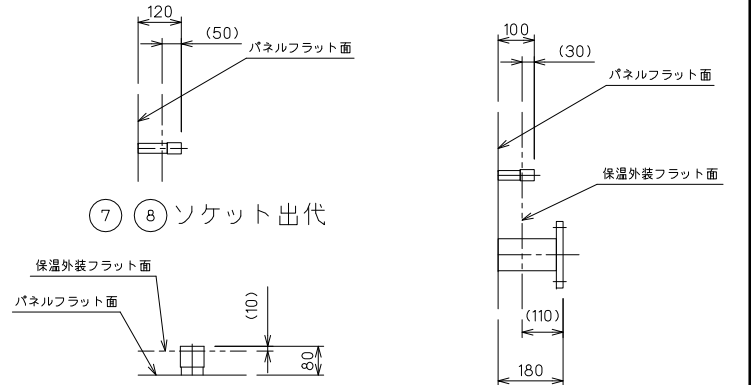
⑦ ⑧ ソケット出代 ⑬ 電極口出代 その他ソケット・フランジ出代
