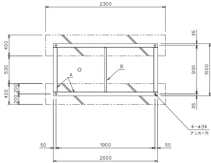
受台伏図
